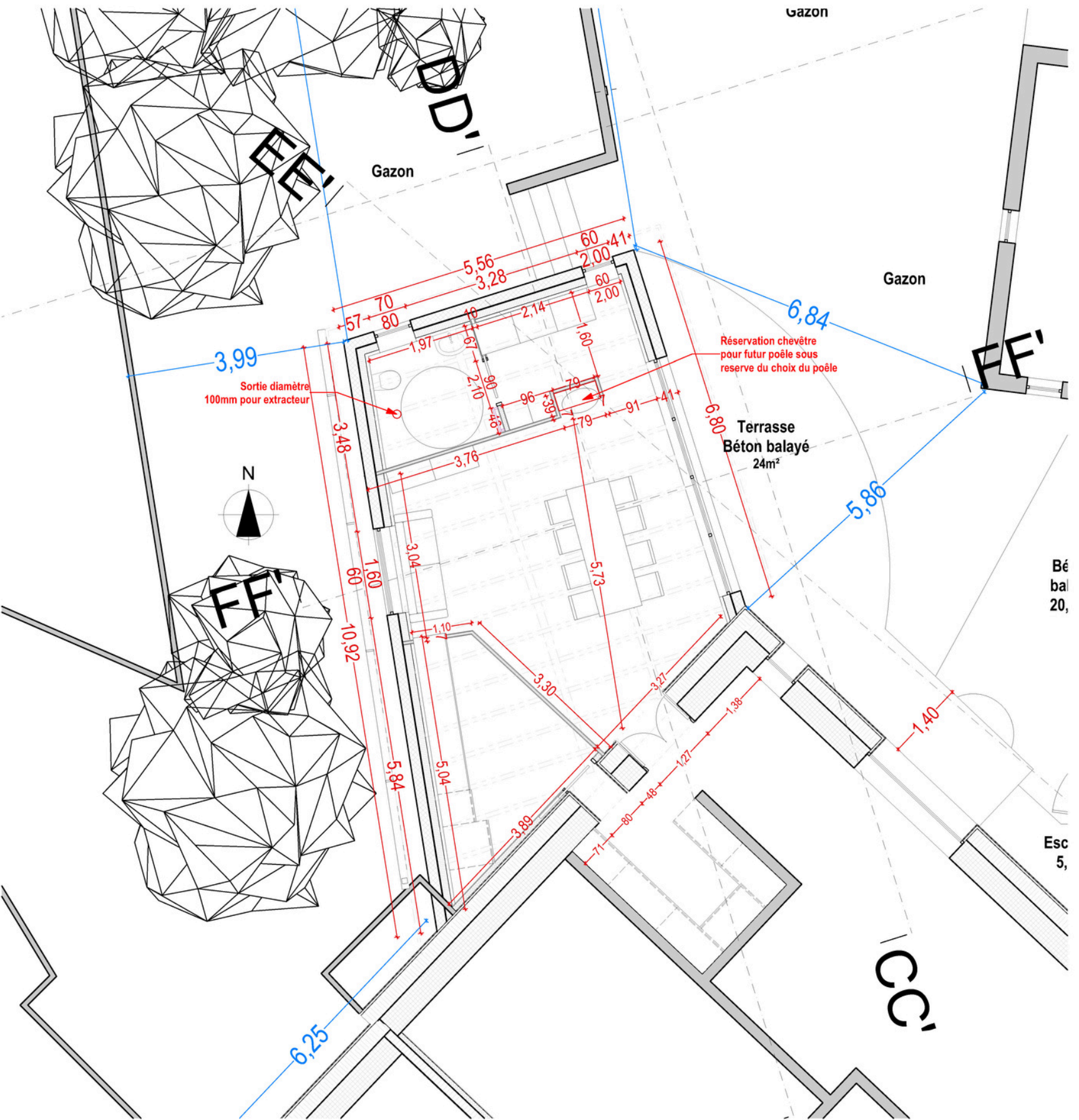
PLAN PLATRIERIE
