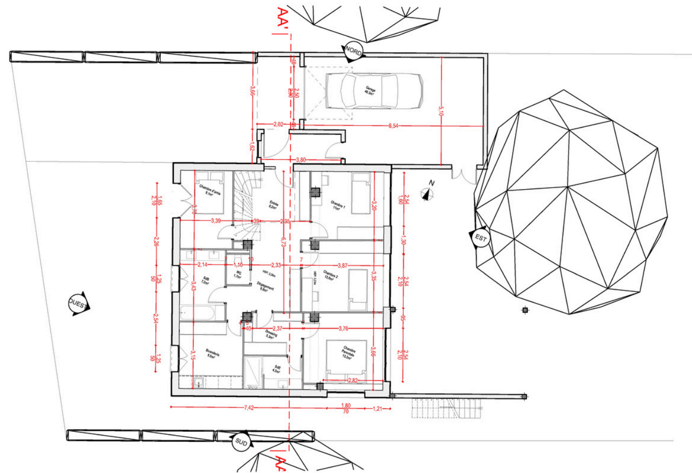
PLAN SOUS-SOL - 1/100
